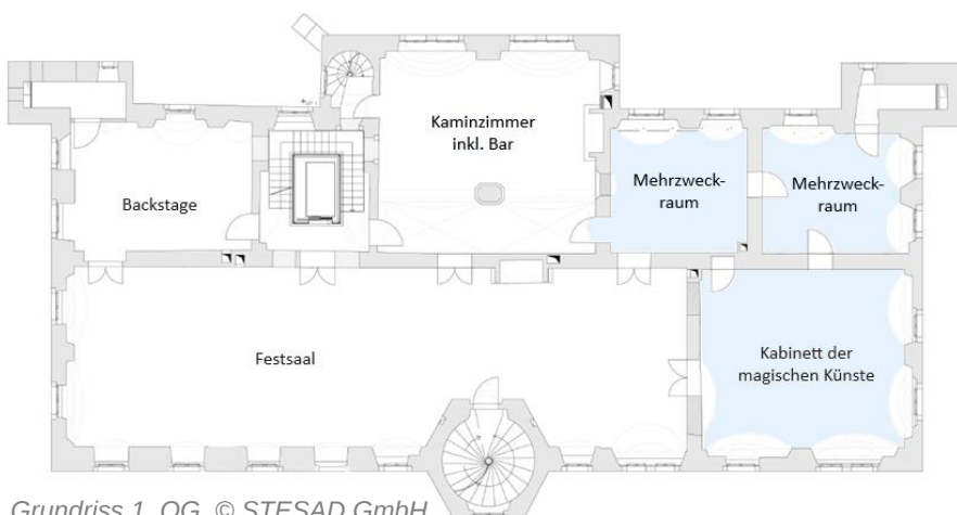
Grundriss 1. OG, © STESAD GmbH
